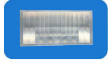
型号：8033 焦距：30 角度：120° 距离：12m 尺寸：33.6×70
